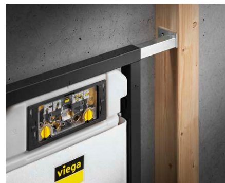
Stenový držiak Prevista Dry: hĺbkové nastavenie bez potreby náradia.
