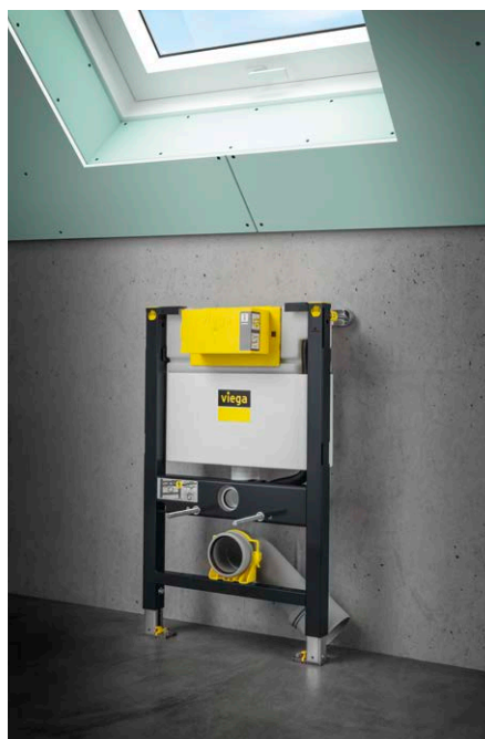
Pre nízke montážne výšky: WC prvok vysoký 820 mm.
